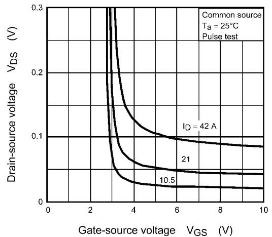
Fig. 8.4 V_{DS} - V_{GS}
